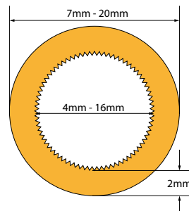
DIREKT ERDVERLEGBARES MIKROROHR
